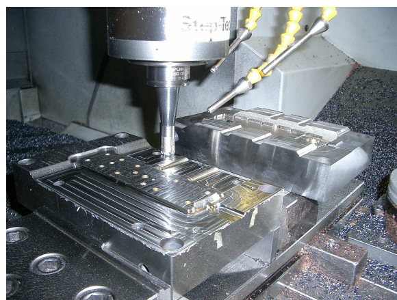
Bearbeitung des Spritzgußeinsatzes mit einem Pokolm Rundplattenwerkzeug.
